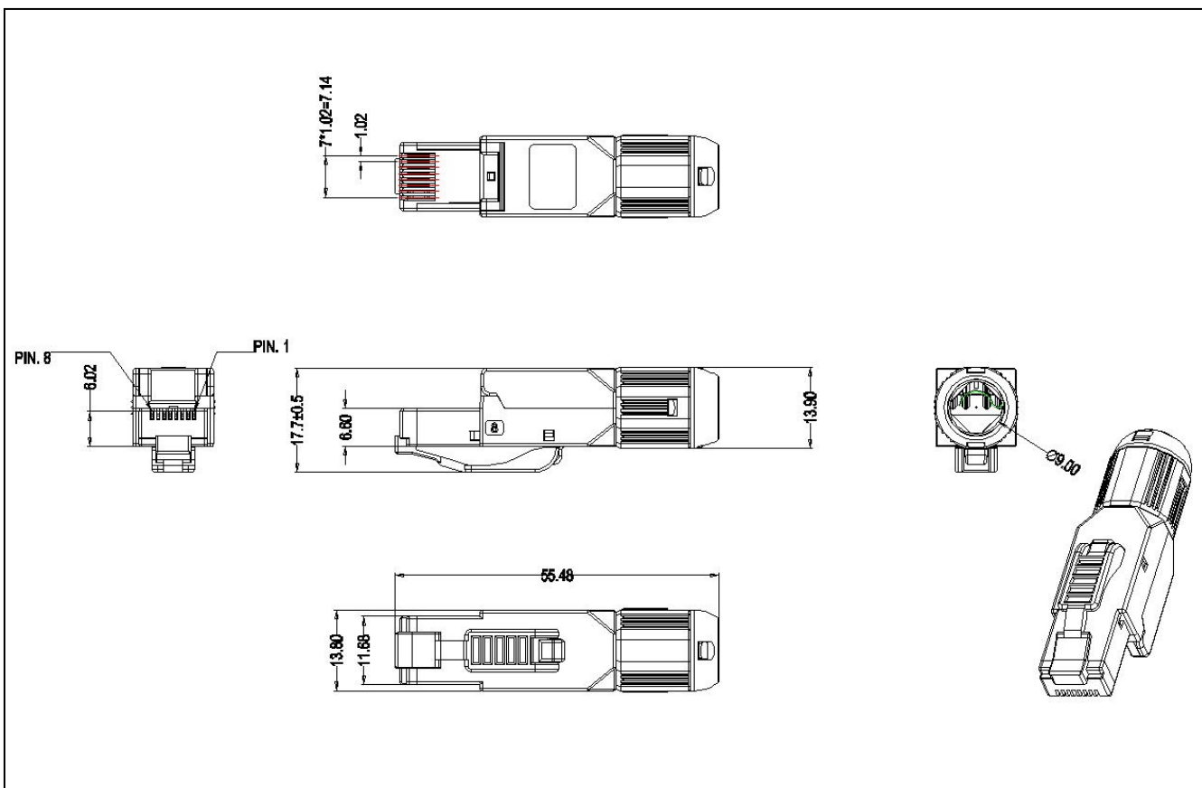
[ 产品结构图 ]
